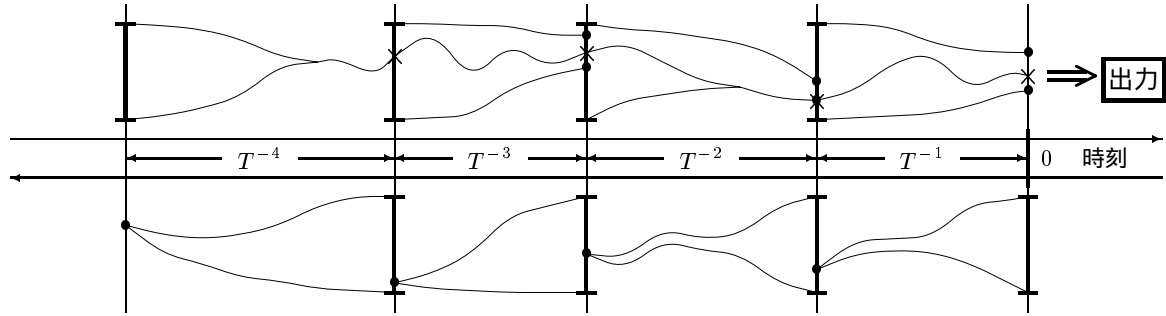
図 4: Twin Run アルゴリズムの概念図
