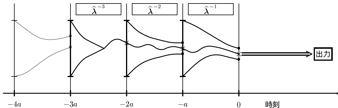
図 2: a 遡る CFTP アルゴリズムの概念図
