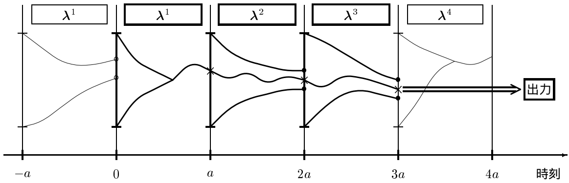
図 3: Read Once アルゴリズムの概念図
