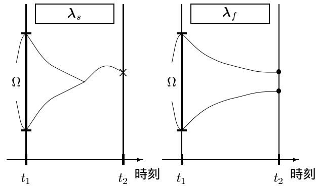
図 1: 時刻 t_1 から時刻 t_2 までの推移の模式図
