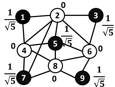
図 1: 最大独立集合問題。●印が最大独立集合の頂点。
