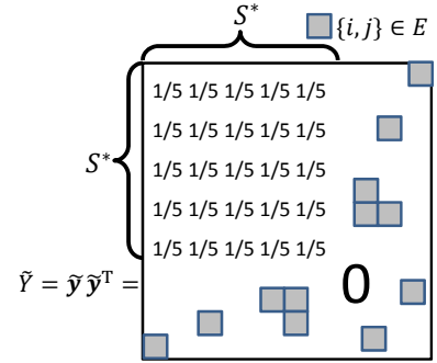
図 2: 図 1 の問題の最適解 \tilde{\mathbf{y}} に対する行列 \tilde{Y} = \tilde{\mathbf{y}}\tilde{\mathbf{y}}^T 。枝集合 E に対応する要素の描画はイメージです。
