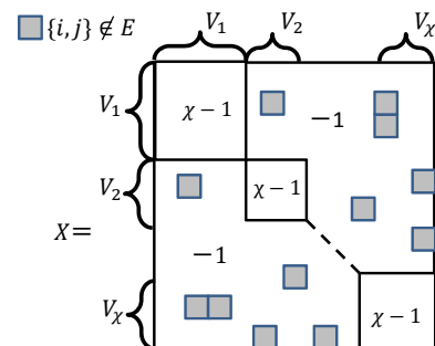
図 3: 行列 X , ただし V_i = \{p \in V \mid c(p) = i\} .
